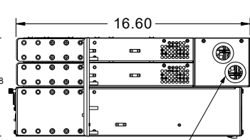
Right Side View Diam. 1.38 (2-places)
